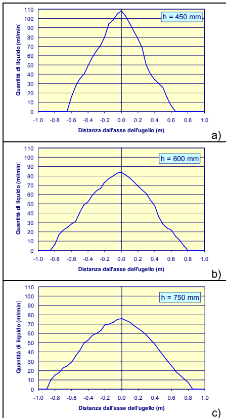
Fig. 2 - Diagrammi di distribuzione ottenuti operando con l'ugello a 0.50 MPa e a diverse altezze rispetto al banco prova.
