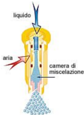
Funzionamento dell'ugello
